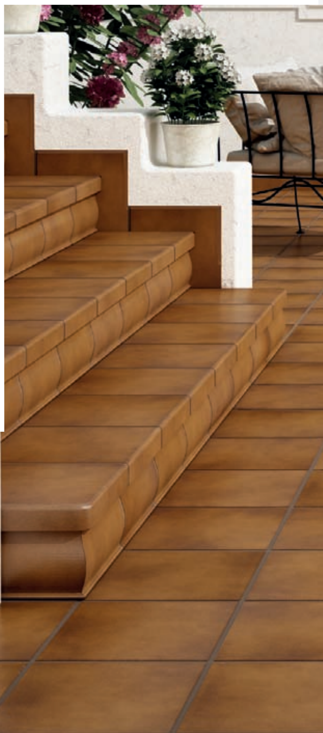
RODAMANTO. BASE 310 x 310. PELDAÑO RECTO, ESQUINA RECTA. TABICA ONDULADA. RODAPIÉ.
